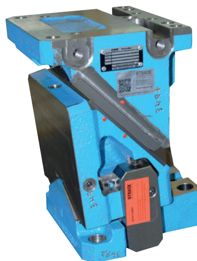
Beispiel 7: Sonderschieber mit verkürzter Bautiefe Example 7: Special cam with reduce installation depth Exemple 7: Coulisseau spécial avec une profondeur d'installation réduite
